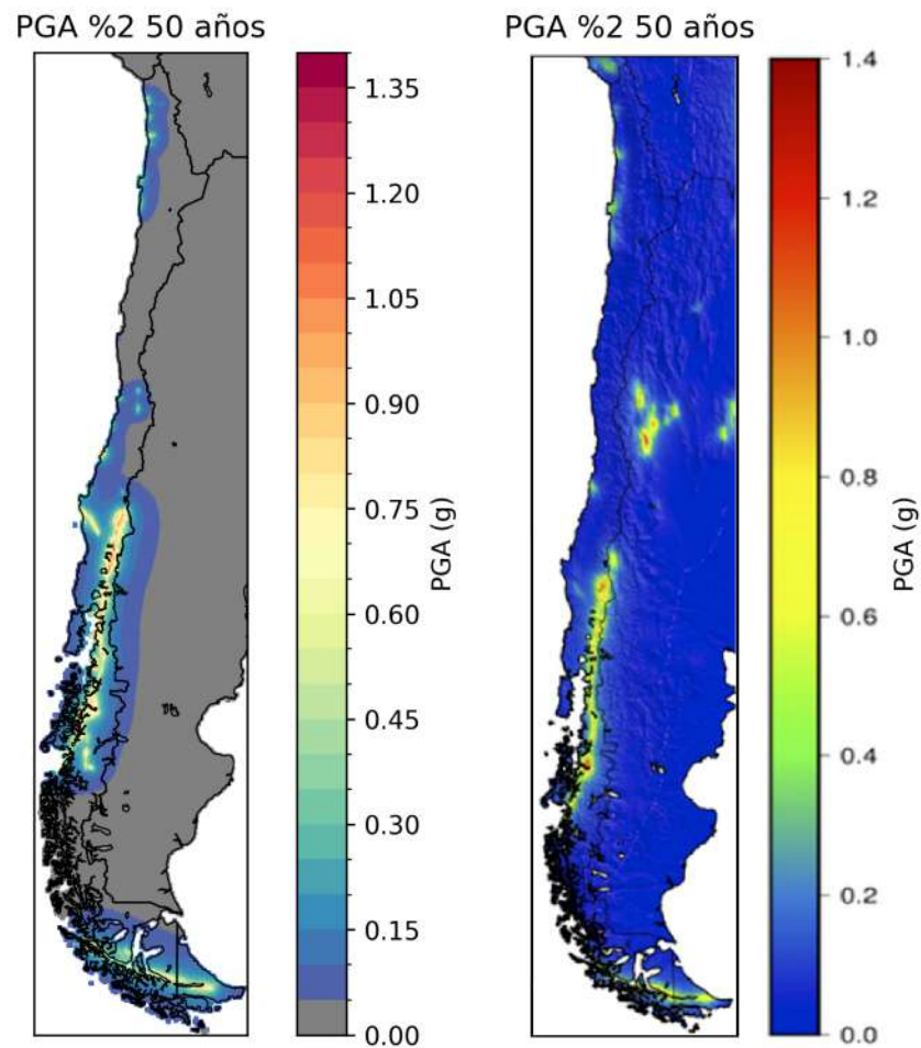
Figura 81. Comparación de mapas de amenaza sísmica de PGA con probabilidad de excedencia 10% en 50 años. Izquierda: Mapa elaborado en este estudio. Derecha: Mapa elaborado para el proyecto SARA (Costa et al., 2020)
