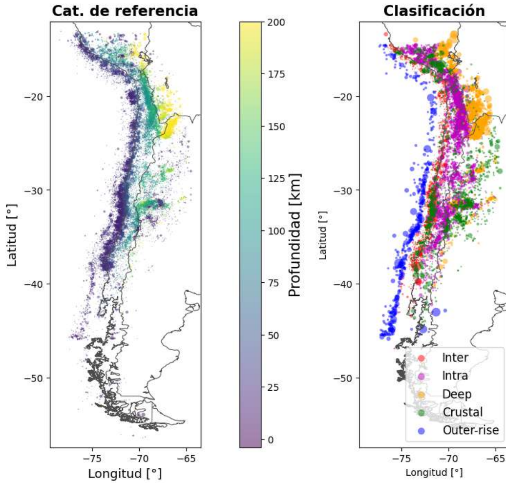
Figura 11. Catálogo de referencia: Izquierda: Distribución de los hipocentros en profundidad. Derecha: Clasificación de la sismicidad.
