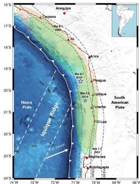
Figura 15. Área de ruptura de los eventos históricos de la zona 1 (Shrivastava et al., 2019)
