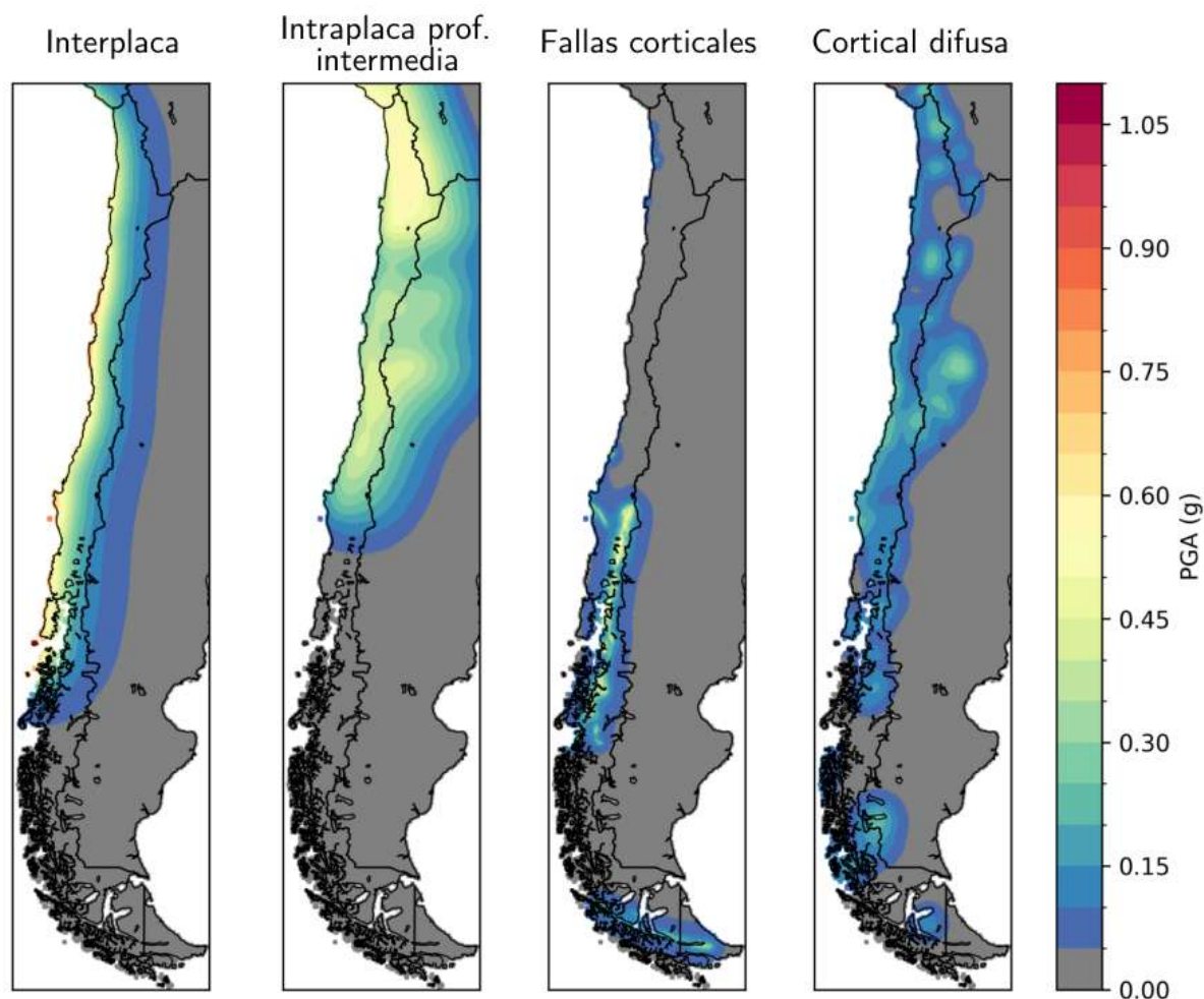
Figura 79. Comparación de mapas de amenaza sísmica de PGA con probabilidad de excedencia 10 % en 50 años.
