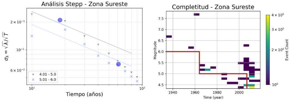
Figura 65. Izquierda: Análisis de Stepp (1972) para el cálculo de completitud del catálogo de la zona Sureste. Derecha: Complejitud del catálogo y densidad de magnitudes con respecto al tiempo.
