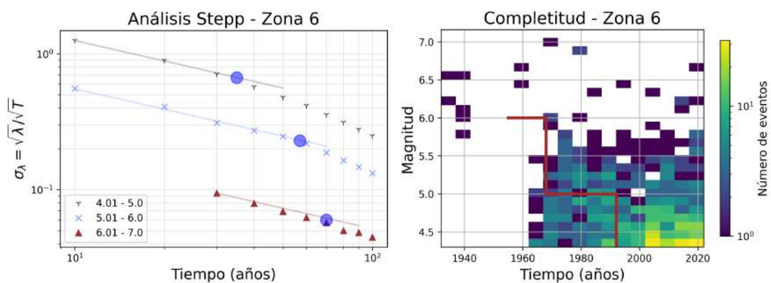
Figura 28. Izquierda: Análisis de Stepp (1972) para el cálculo de completitud del catálogo de la zona 6. Derecha: Completitud del catálogo y densidad de magnitudes con respecto al tiempo.
