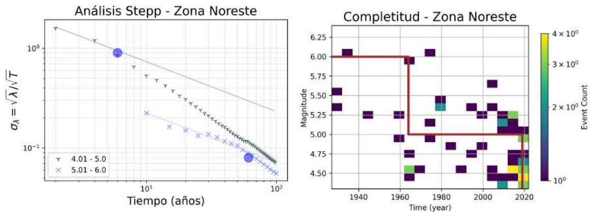
Figura 57. Izquierda: Análisis de Stepp (1972) para el cálculo de completitud del catálogo de la zona Noreste. Derecha: Completitud del catálogo y densidad de magnitudes con respecto al tiempo.
