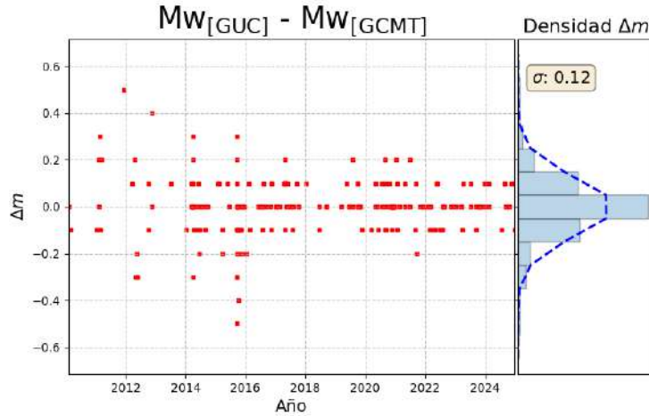
Figura 6. Distribución de la diferencia entre los reportes Mw(GUC) y Mw(GCMT)
