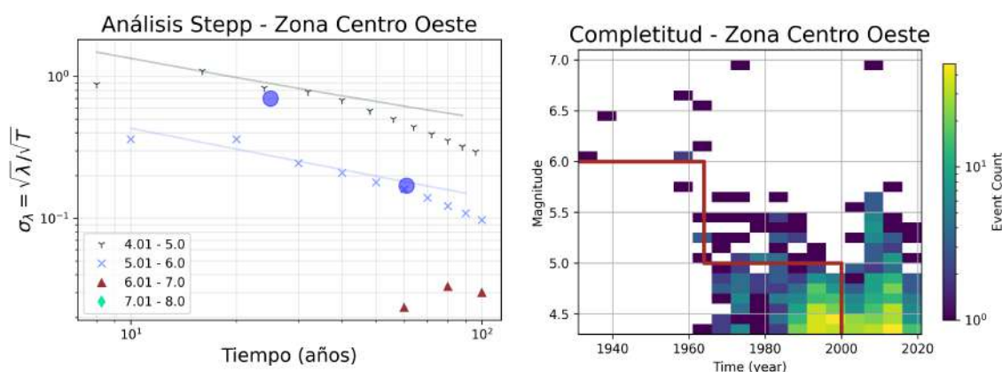
Figura 59. Izquierda: Análisis de Stepp (1972) para el cálculo de completitud del catálogo de la zona Centro Oeste. Derecha: Completitud del catálogo y densidad de magnitudes con respecto al tiempo.
