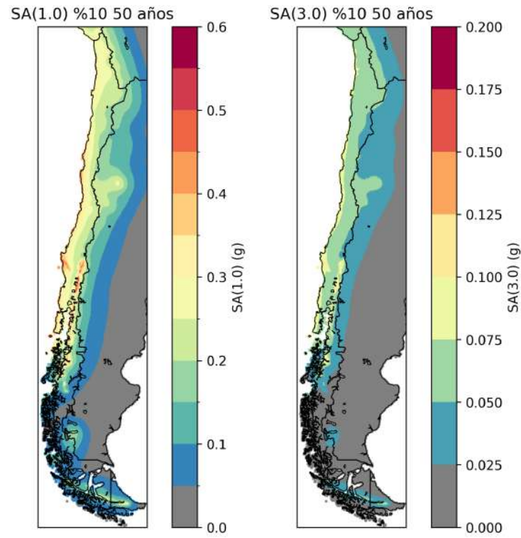
Figura 76. Mapa de amenaza para SA(1.0) y SA(3.0) con probabilidad de excedencia del 10% en 50 años para Chile continental
