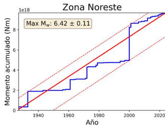
Figura 58. Liberación de momento sísmico acumulado en Zona Noreste
