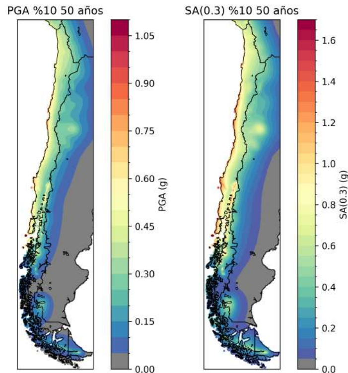
Figura 75. Mapa de amenaza para PGA y SA(0.1) con probabilidad de excedencia del 10 % en 50 años para Chile continental
