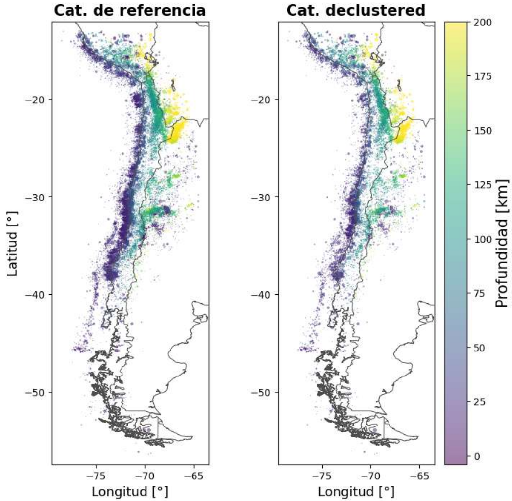
Figura 12. Izquierda: Catálogo de referencia. Derecha: Catálogo depurado (post declustering)
