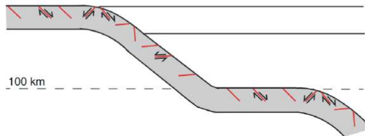
Figura 71. Esquema de planos de falla de eventos intraplaca para Sudamérica descritos en Warren (2014). El ángulo de manteo de los eventos subverticales y subhorizontales se encuentran definidos principalmente por la superficie superior de la placa subductante.
