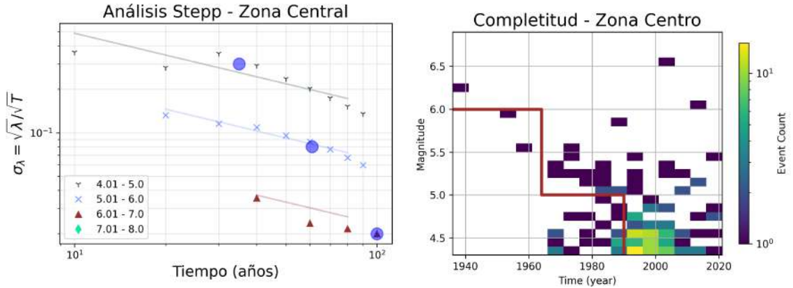
Figura 61. Izquierda: Análisis de Stepp (1972) para el cálculo de completitud del catálogo de la zona Central. Derecha: Complejitud del catálogo y densidad de magnitudes con respecto al tiempo.
