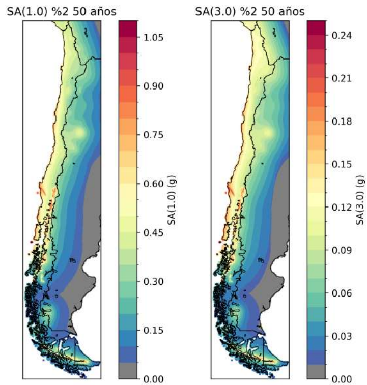
Figura 78. Mapa de amenaza para SA(1.0) y SA(3.0) con probabilidad de excedencia del 2% en 50 años para Chile continental
