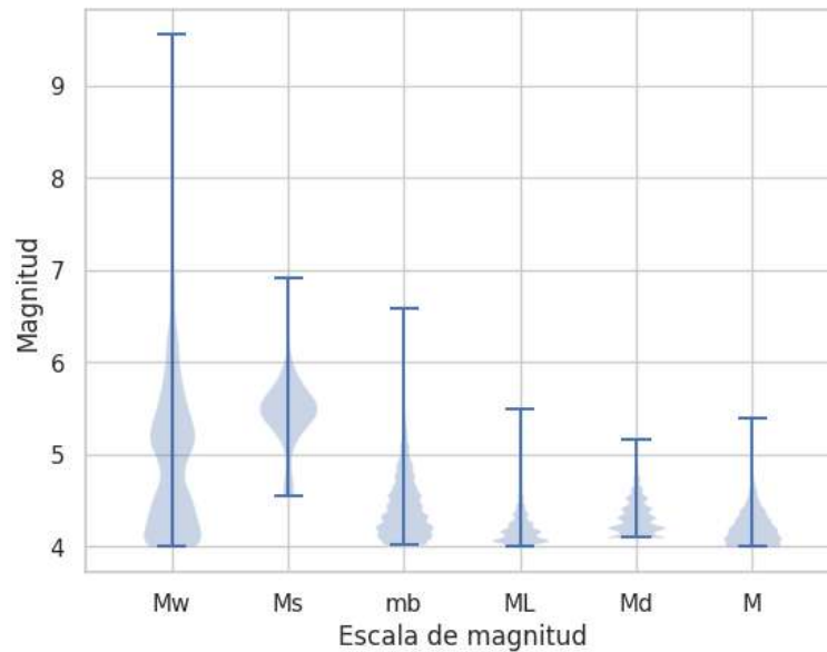
Figura 8. Gráfico de violín para las escalas de magnitud
