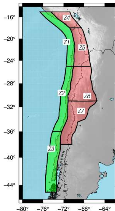
Figura 13. Zonificación de las fuentes de subducción propuesta por Martin (1990)
