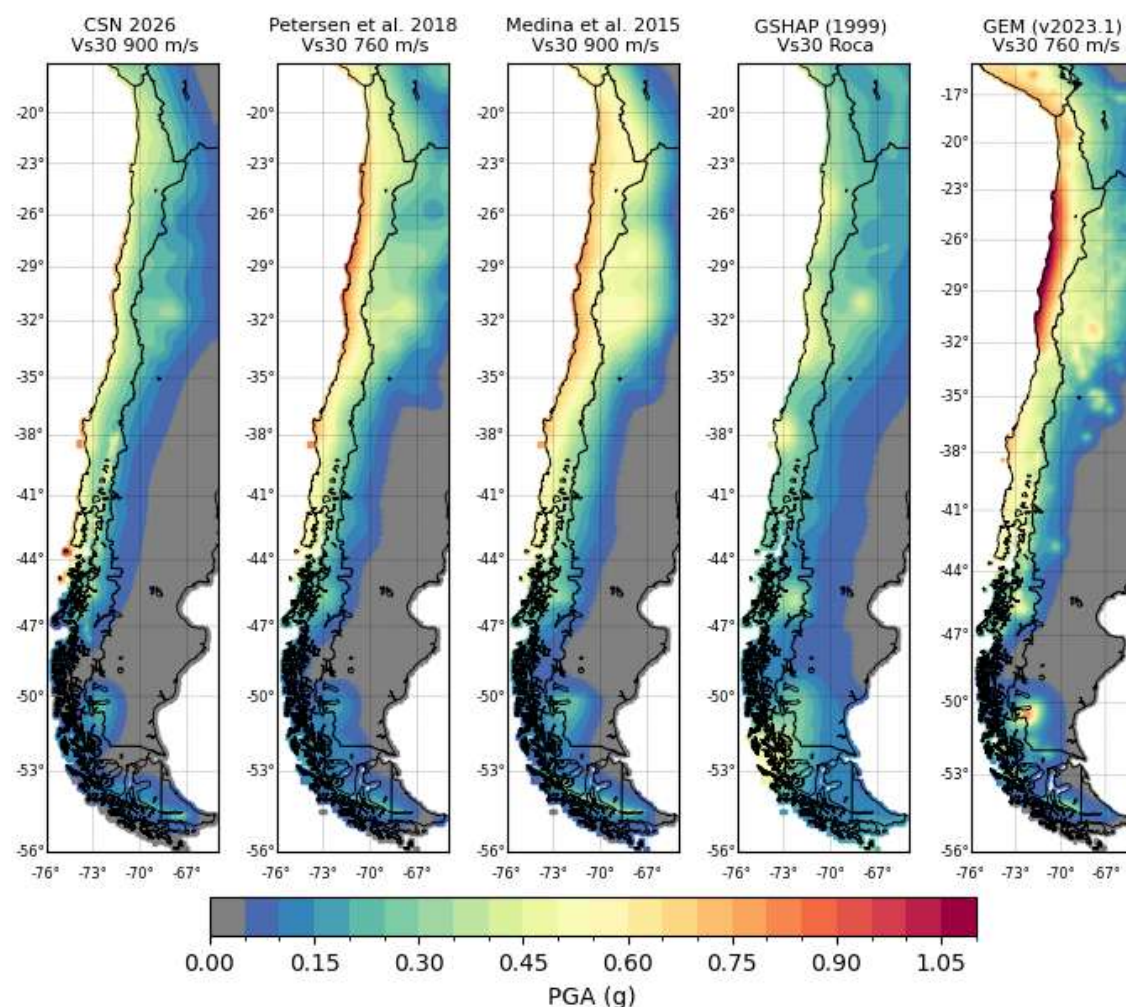
Figura 80. Comparación de mapas de amenaza sísmica de PGA con probabilidad de escendencia 10% en 50 años.
