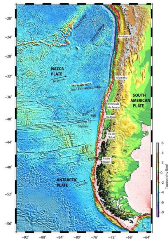
Figura 1. Configuración geodinámica (Contreras-Reyes et al., 2018)
