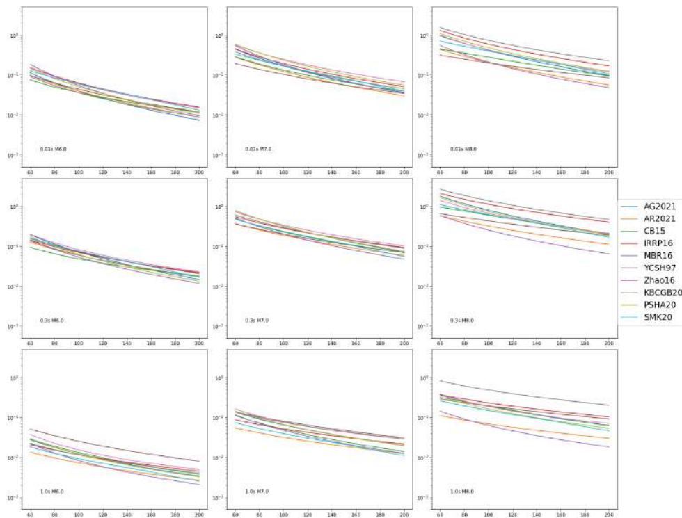
Figura 46. Gráficos de grillas distancia vs respuesta para sismos intraplaca.
