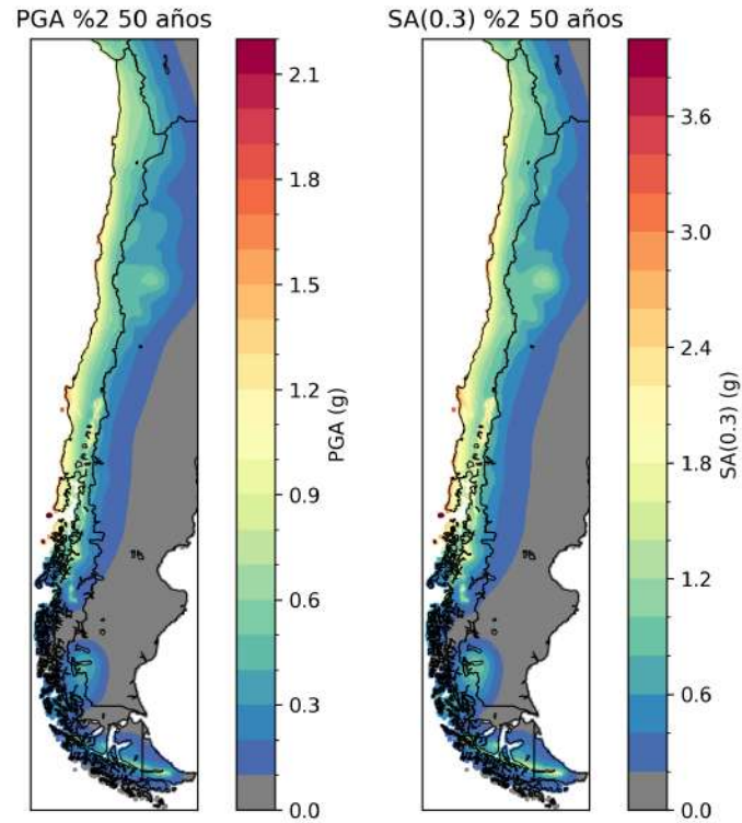
Figura 77. Mapa de amenaza para PGA y SA(0.1) con probabilidad de excedencia del 2% en 50 años para Chile continental
