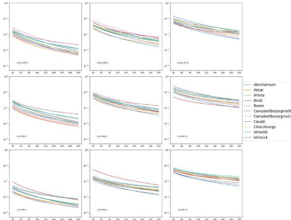
Figura 50. Gráficos de grillas distancia vs respuesta para sismos corticales.
